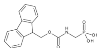
1. AMPA-FMOC
